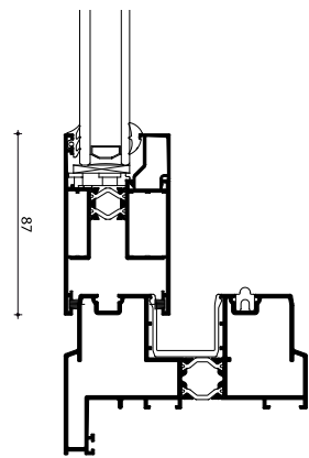
duorail
